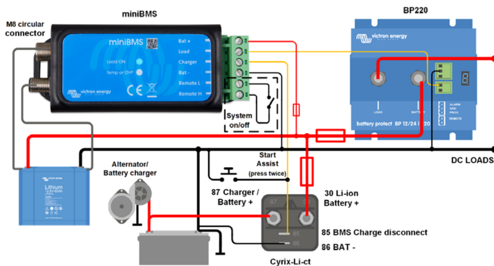
Bild 2: Användningsexempel för ett fordon eller en båt, med systemets av/på-brytare mellan H
